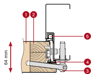
OCELOVÁ ZÁRUBŇA
