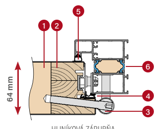
HLINÍKOVÁ ZÁRUBŇA
