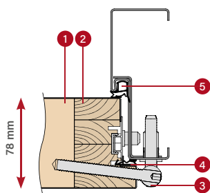
OCELOVÁ ZÁRUBŇA
